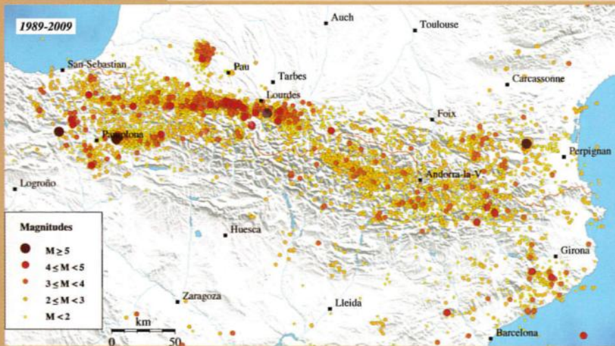
Sismicité dans les Pyrénées de 1989 à 2009 – Observatoire Midi-Pyrénées
