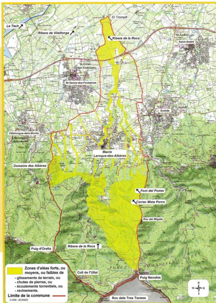
Aléas mouvements de terrain du PPR.
